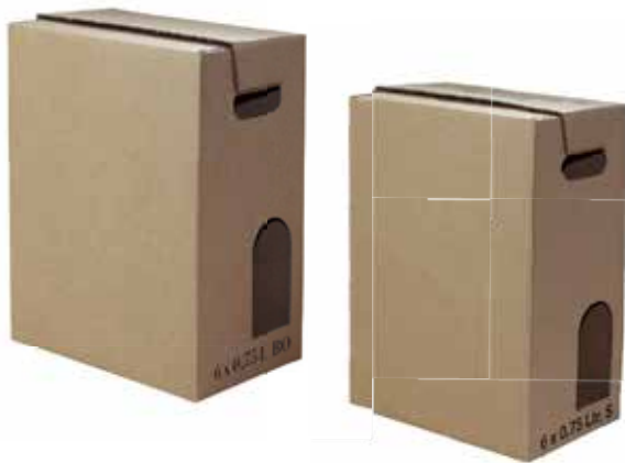
Faltbodenschachtel 6 x 0,75 ltr. Schlegel mit Automatikboden, stehend, mit Fenster I-Maße: 228 x 152 x 330 mm, 800 St./Pal.
